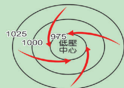
北半球氣旋
