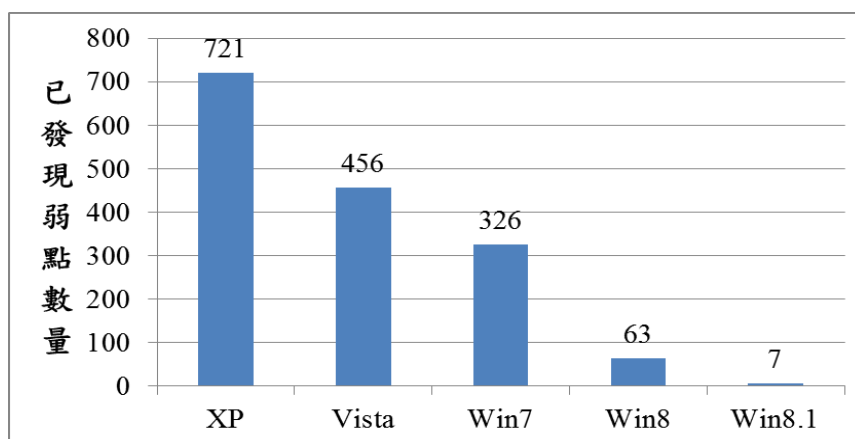
資料來源：CVE Details 弱點資料庫[4]
