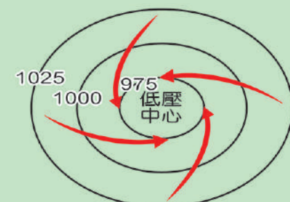
北半球氣旋
