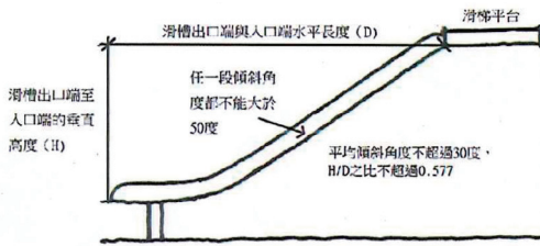
圖 3-48 滑槽平均傾斜角度之設計
