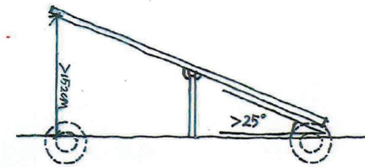
圖 3-70 槓桿式跳跳板之座位與水平線間的傾斜夾角不可超過 25 度；槓桿式跳跳板的座位距離防護鋪面的高度小於 152 公分。
