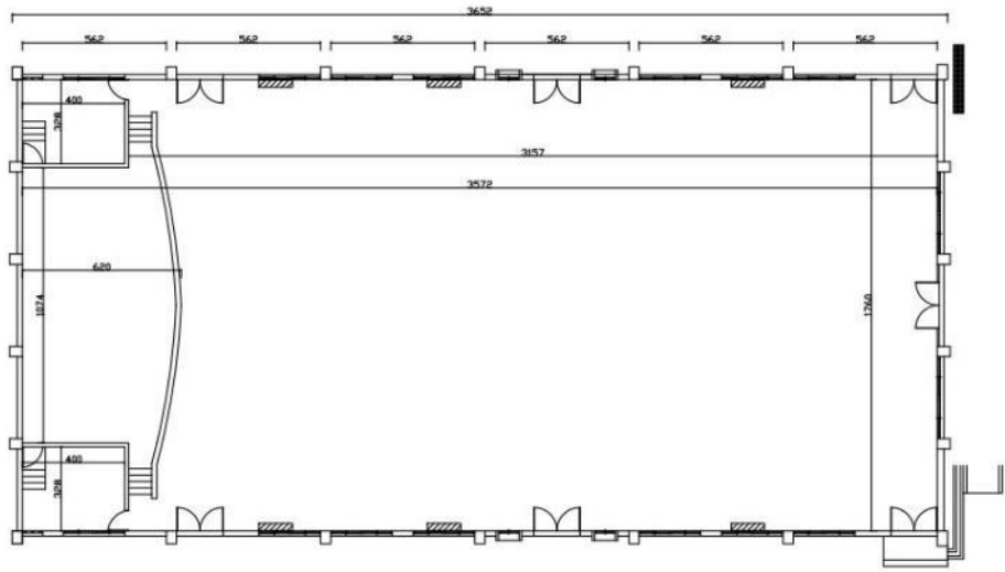
一層平面圖 S: 1/100
