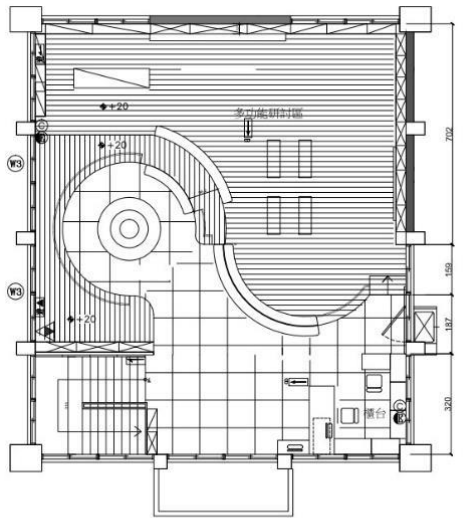
圖書館二樓平面圖 S:1/100
