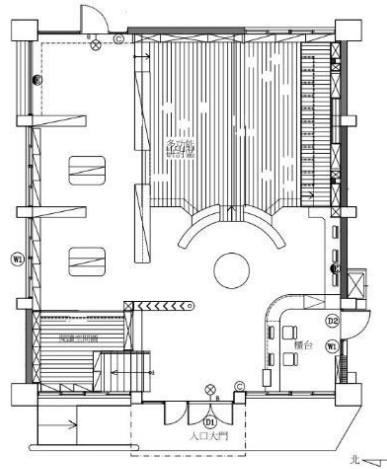
圖書館一樓平面圖 S:1/100
